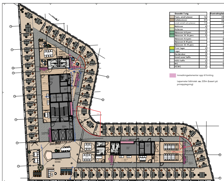
Møbleringsplan nivå 7.
